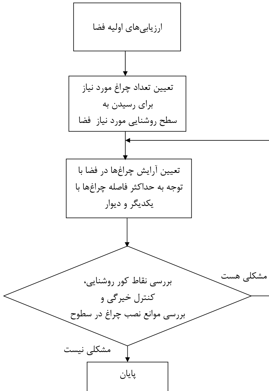
شکل (۱-۲). روند نمای مراحل طراحی سیستم روشنایی در فضاهای داخلی
